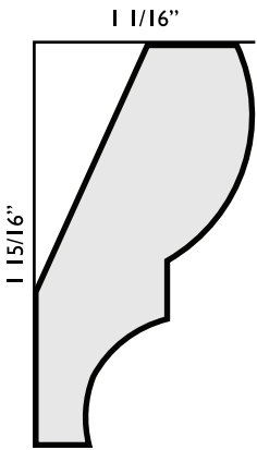
P256 1 1/16" x 2 1/4" CROWN/CORNICE
